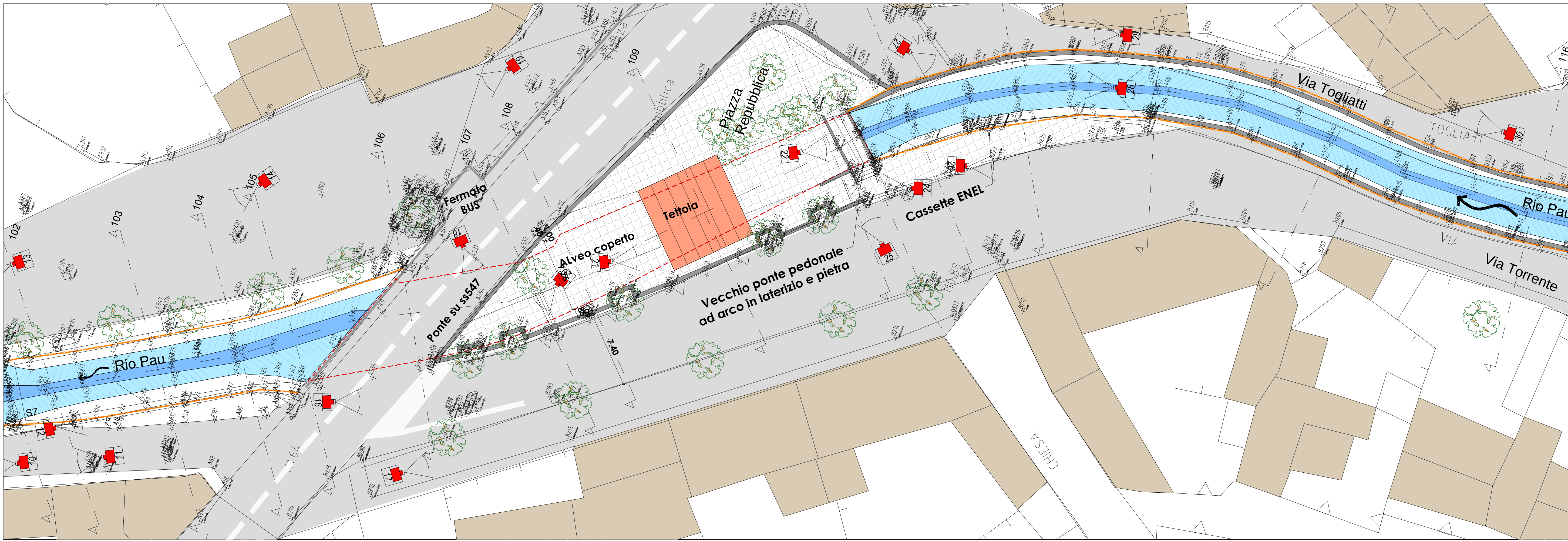
STATO ATTUALE : PLANIMETRIA AREA DI INTERVENTO - scala 1 : 200
