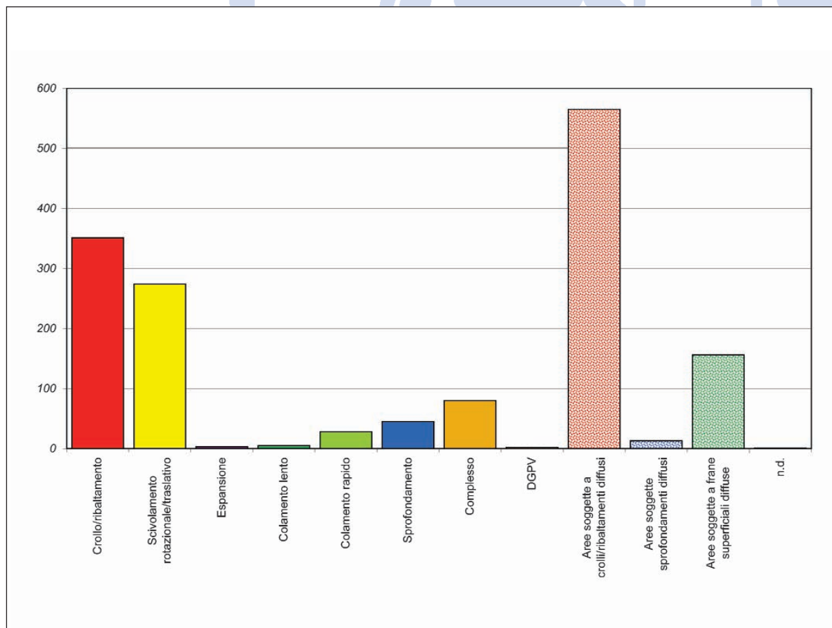
Figura 7: Numero di frane per tipologia di movimento. Si evidenzia una preponderante distribuzione e frequenza di frane ascrivibili alla tipologia di movimento “Aree soggette a crolli e ribaltamenti diffusi”; segue, in ordine di frequenza, la tipologia di movimento franoso “crollo-ribaltamento” e “scivolamento rotazionale e traslattivo”; numericamente minori gli altri movimenti, fra cui le tipologie “aree soggette a frane superficiali diffuse” e “complesso” risultano significative.
