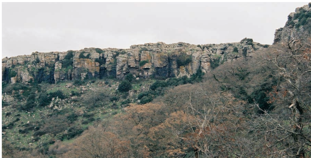
Comune di Bessude (SS) – Cornici Basaltiche con fratturazione sub-verticale. Frane di crollo diffuse, con distacchi di blocchi dalle cornici basaltiche, imputabili alle alterazioni determinate dagli agenti atmosferici, impostate in giunti preesistenti.
