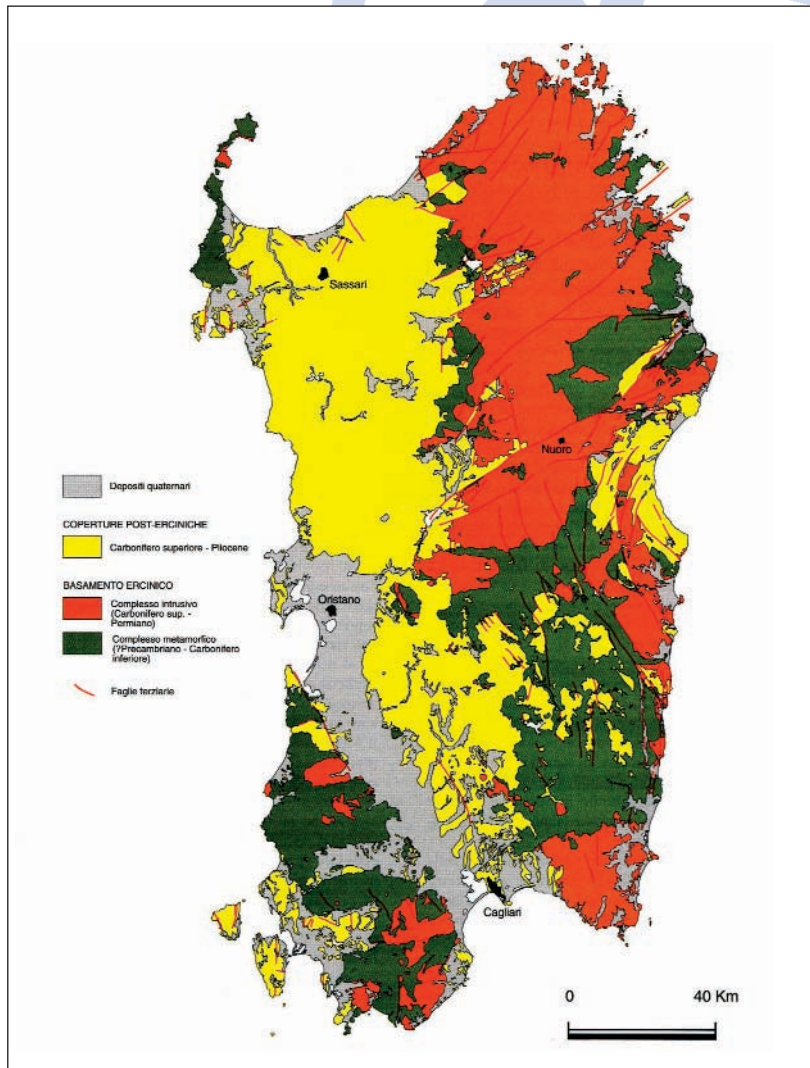
Figura 4: Principali complessi geologici della Sardegna 2
