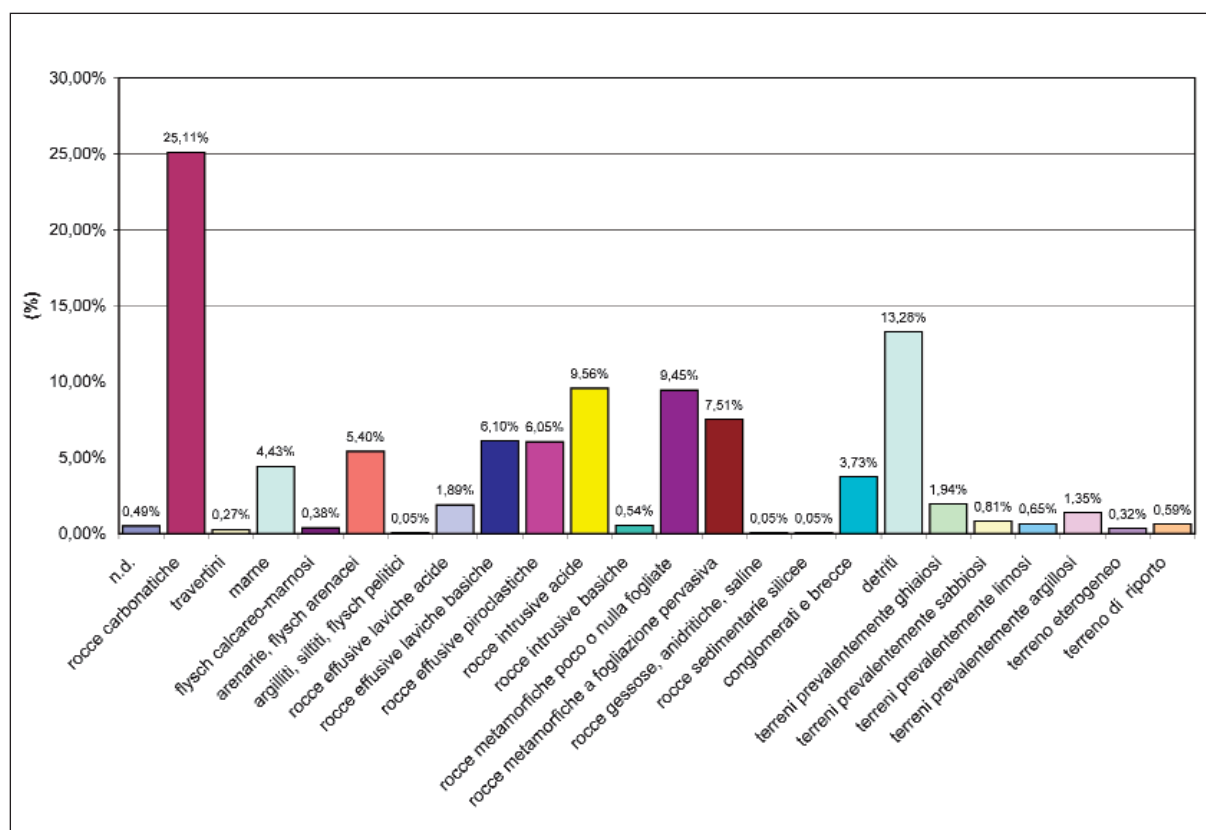
Figura 11: Franosità percentuale per classi litologiche.
