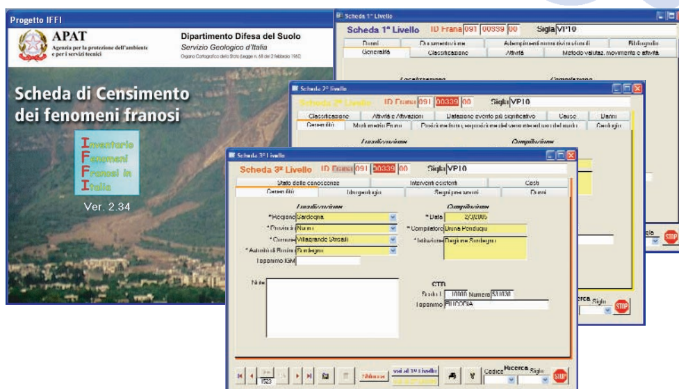
Figura 2: Database dei fenomeni franosi.
