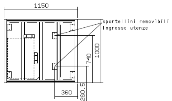
Dettaglio piattaforma
